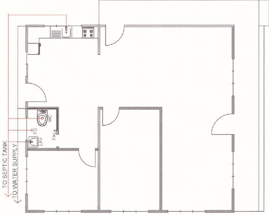
PLUMBING LAYOUT SCALE: 1:100
